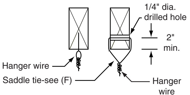
(D) At bottom of joist
