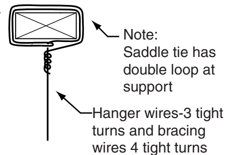
(F) Typ. saddle tie
